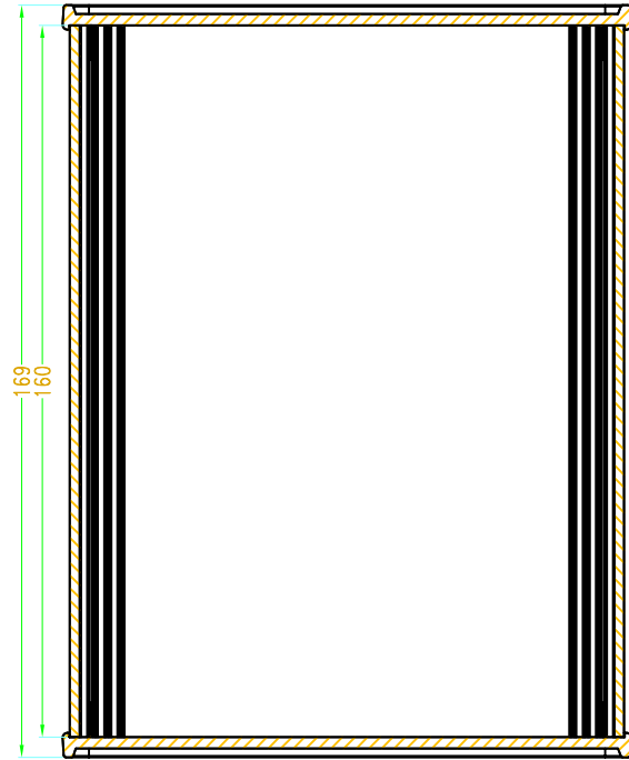
SEC A-A
