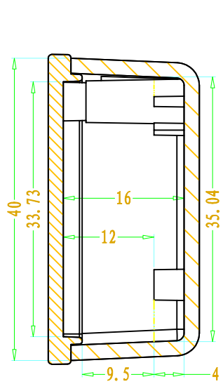
SEC A-A
