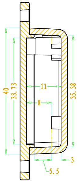
SEC A-A
