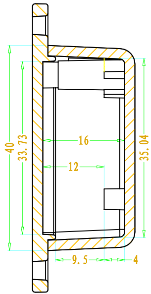
SEC A-A
