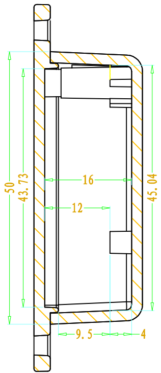
SEC A-A
