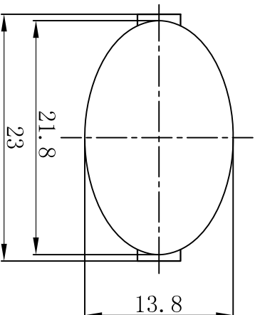
安装面板尺寸 PANEL CUT-OUT
